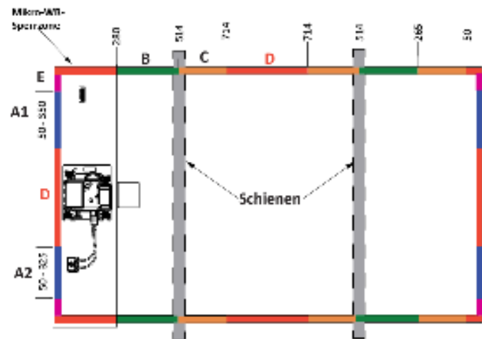
Abb. 1: Mit Schienenunterstützung
