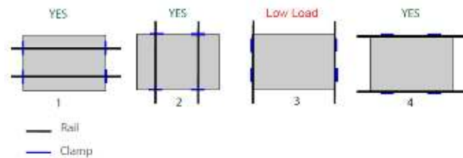
図 3. 架台の構成
